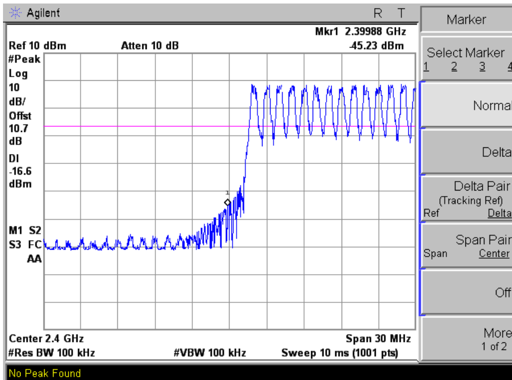
– Band edge lower side (GFSK) Hopping On–
