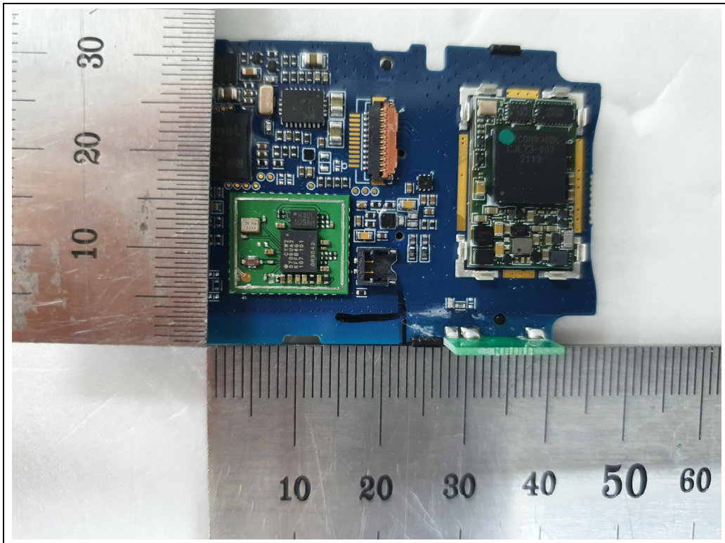
<BT Module>
