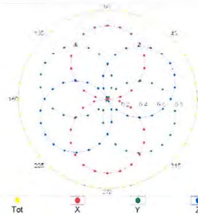
f=1800 MHz,R22
