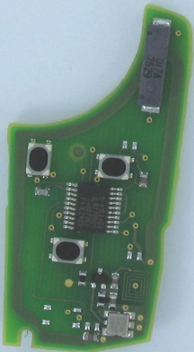
3 Button 314.90MHz
