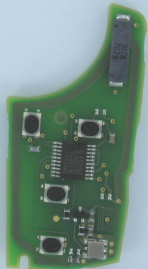
4 Button 314.90MHz
