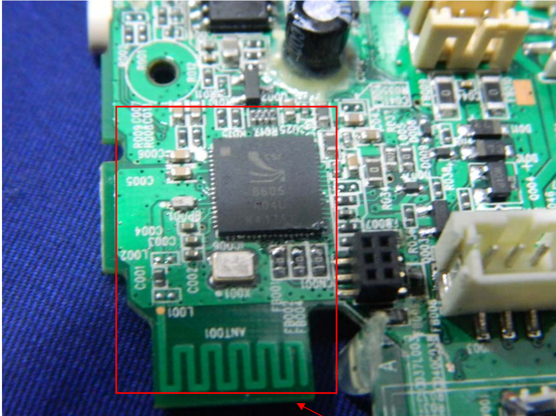
Bluetooth module
