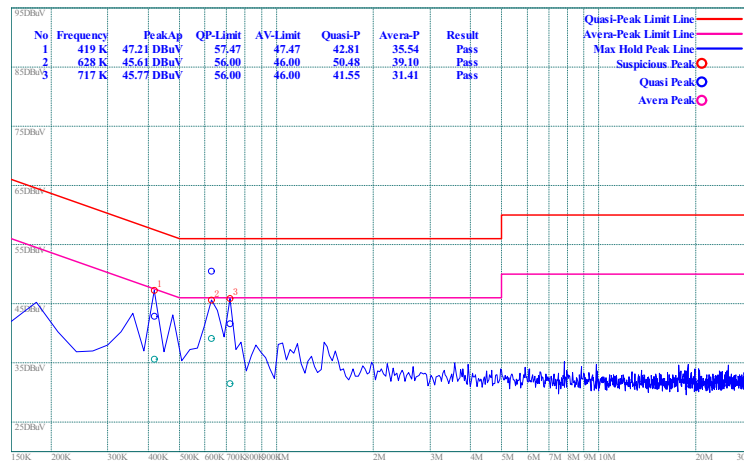
(Plot B: N Phase)
