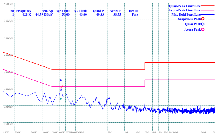
(Plot A: L Phase)
