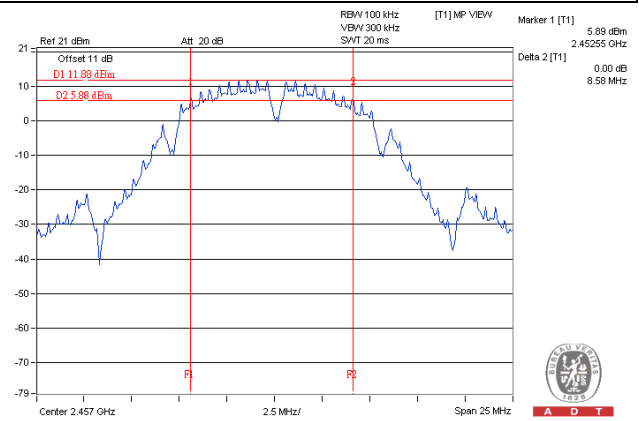
802.11n (HT20) / Chain 1 : CH10
