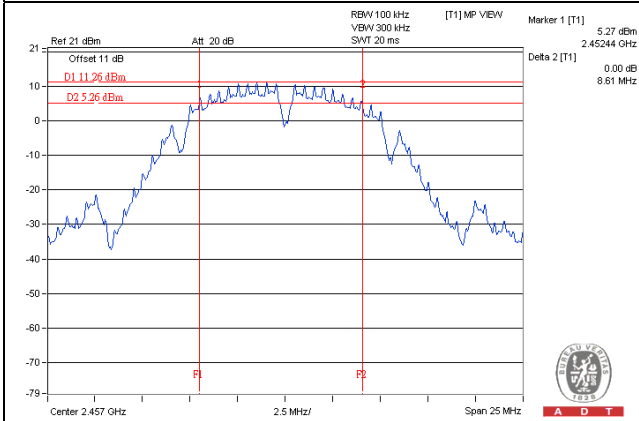
802.11g / Chain 1 : CH10
