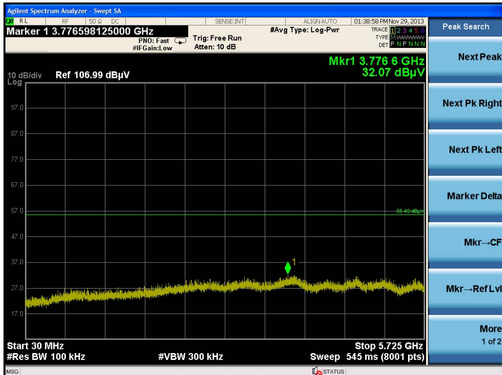
Plot on Configuration IEEE 802.11n MCS0 20MHz / CH 165 / 30MHz~5725MHz (down 30dBc)
