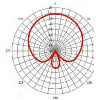
Vertical (ETSI)
