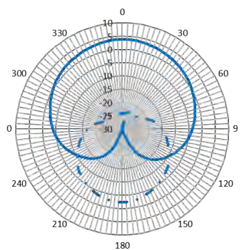
Vertical (ETSI)
