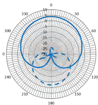
Horizontal (ETSI)
