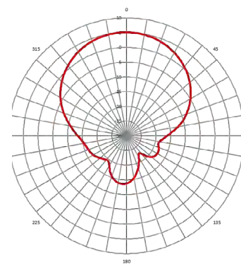
Vertical (ETSI)
