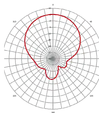
Vertical (ETSI)
