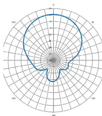
Horizontal (ETSI)
