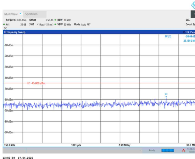
Band41-20MHz-QPSK-39750-1RB#0-Range2:0.15~30MHz
