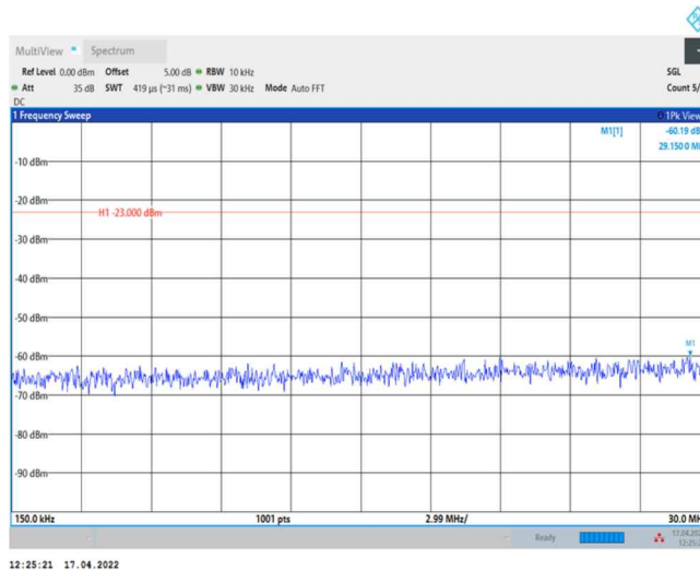
Band4-20MHz-QPSK-20050-1RB#0-Range2:0.15~30MHz
