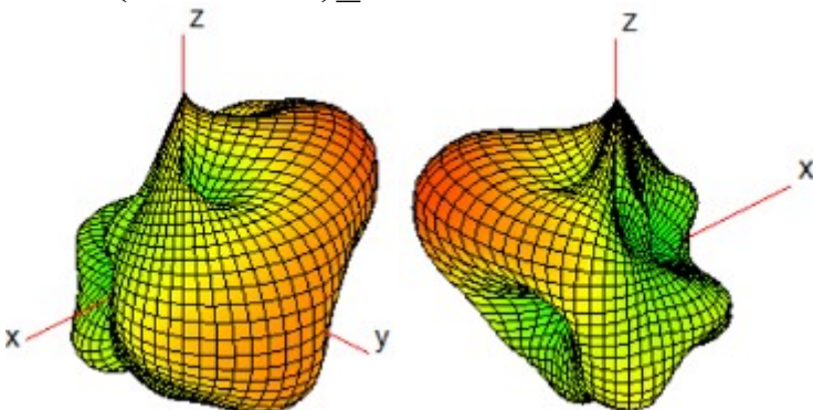
Ant 8(WiFi1/BT)_6200MHz
