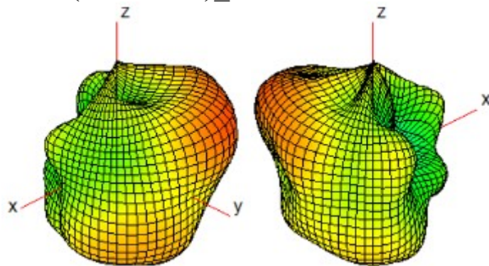
Ant 8(WiFi1/BT)_7000MHz
