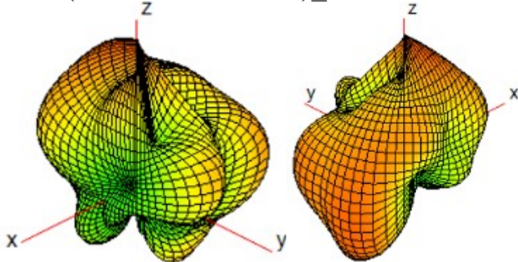
Ant 8(WiFi1/BT)_2450MHz
