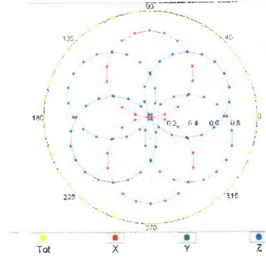
f=1800 MHz,R22
