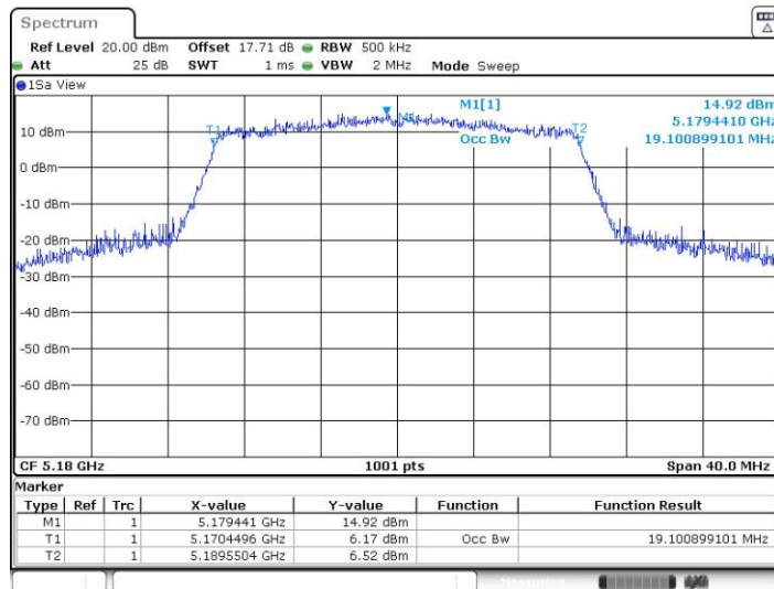
11AX20MIMO_Ant2_5180
