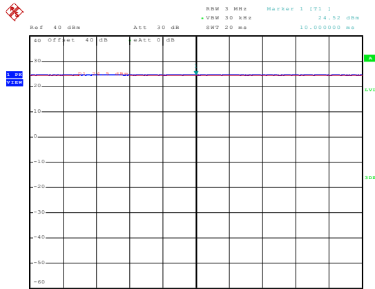
1900MHz - CW
