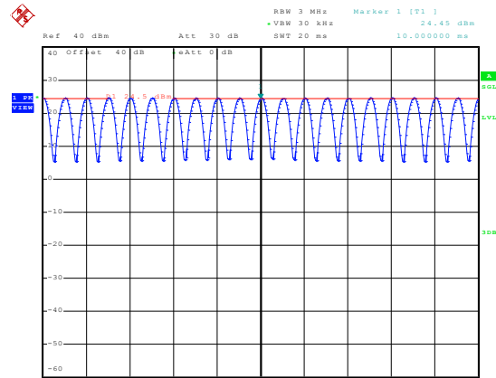
1900MHz - 80% AM
