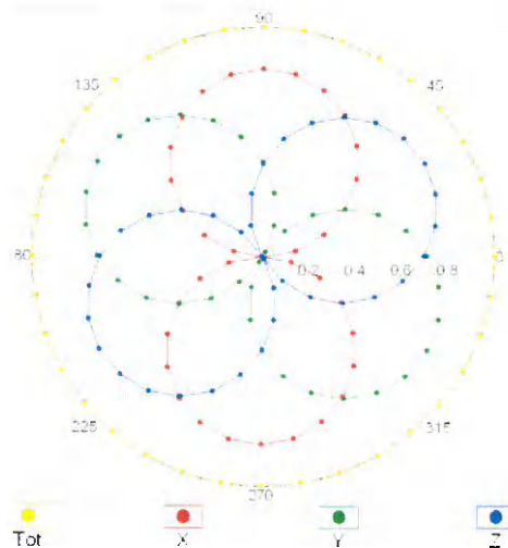
f=1800 MHz.R22
