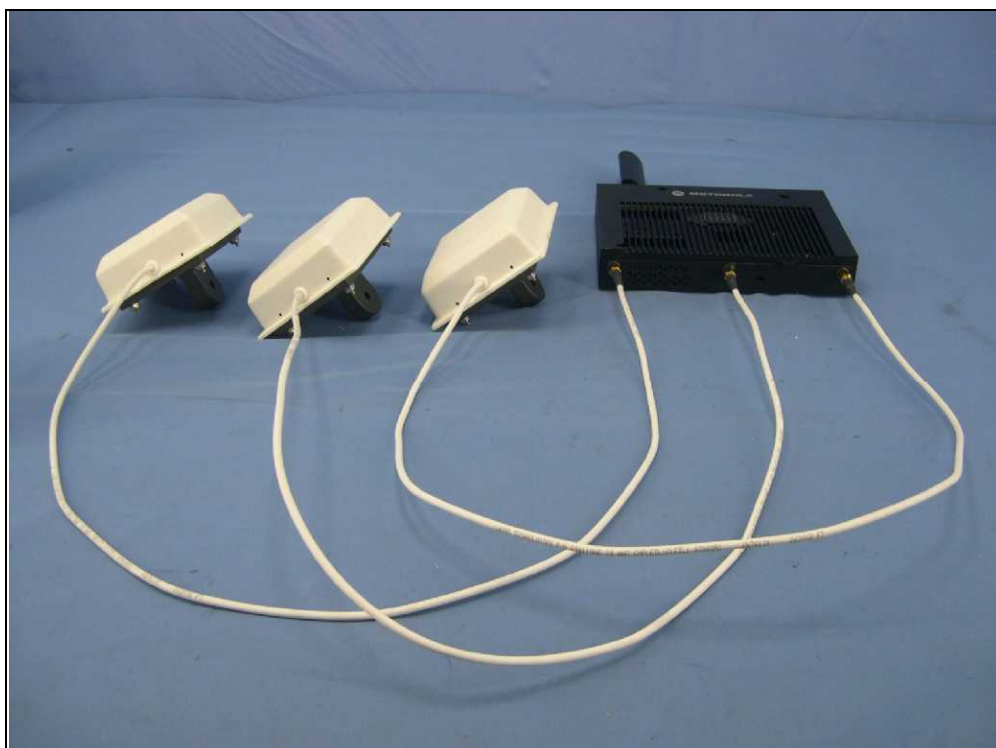
Antenna 5: ML-5299-WPNA1-01R
