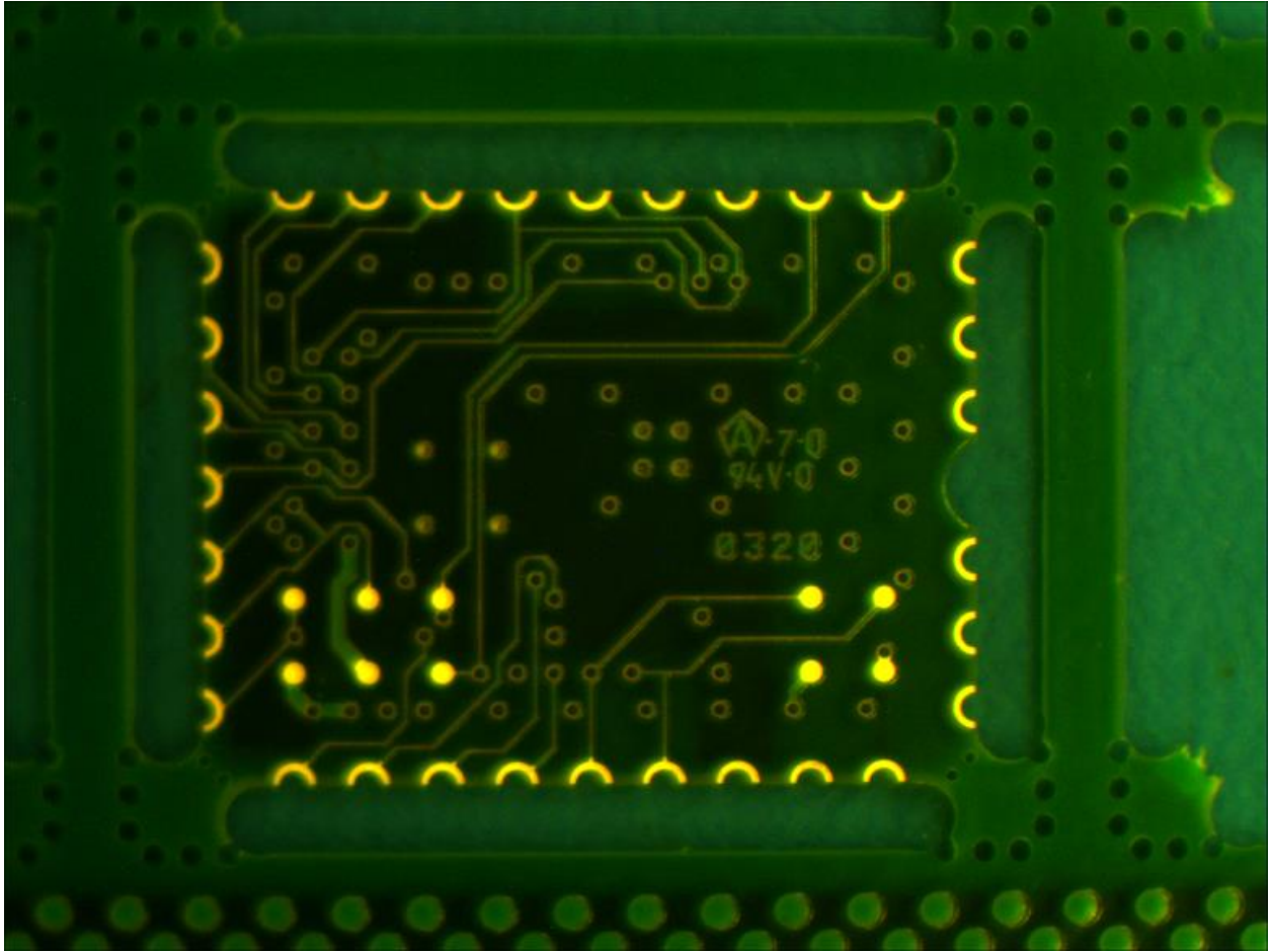
Payload Module Bottom
