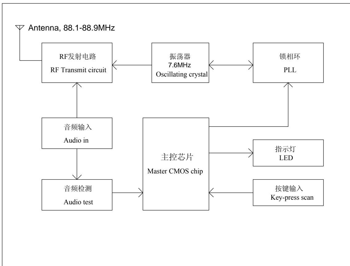
电路方框图 Block Diagram
