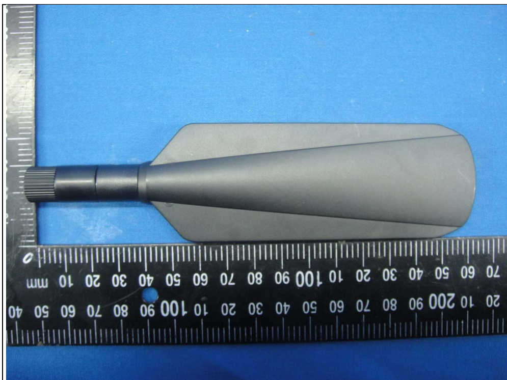
LTE Antenna (No. 2)
