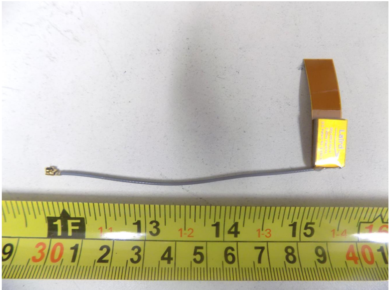
Figure 5: BLE antenna
