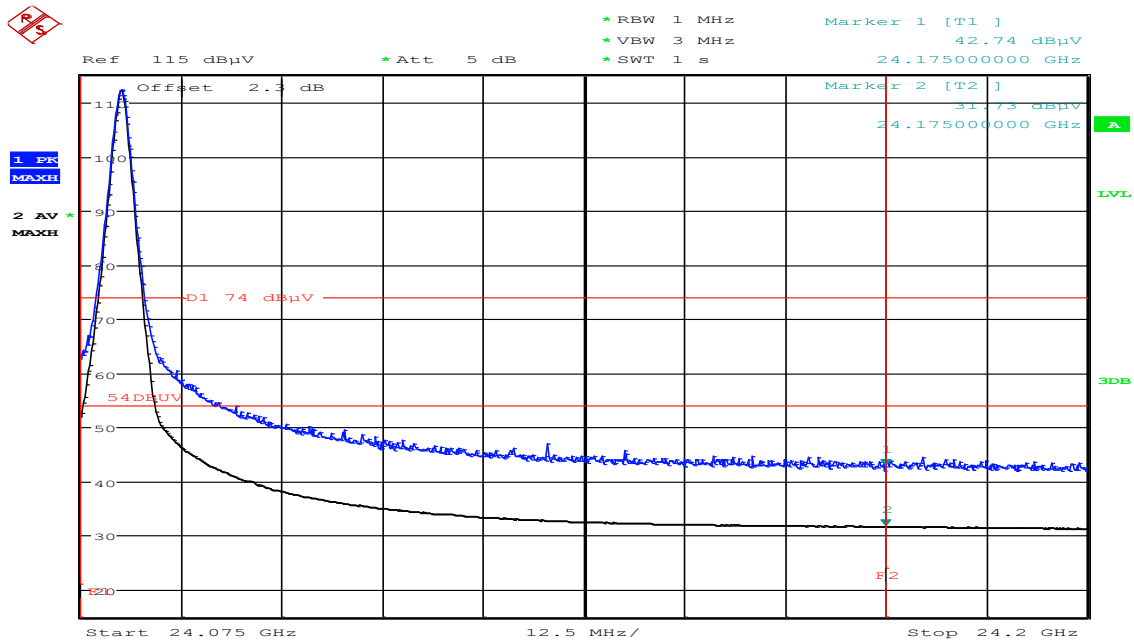
Plot 9: Band edge compliance, Upper edge
