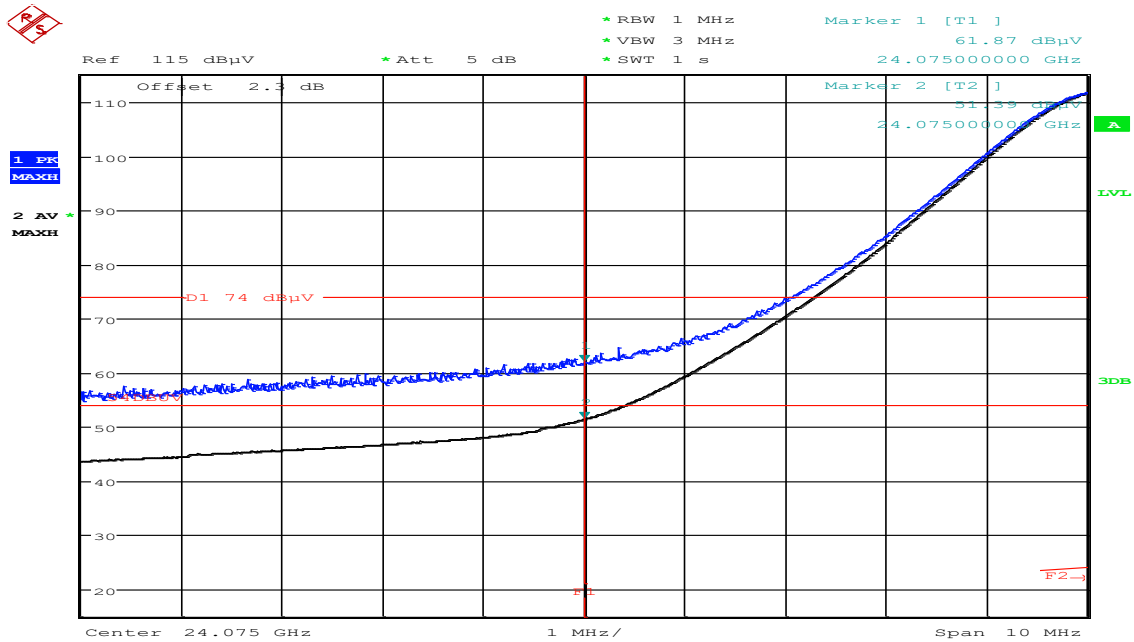
Plot 8: Band edge compliance, Lower edge
