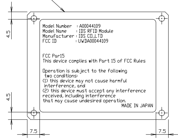
ラベル貼りつけ位置図 IDS RFID Module カバーの上にラベル貼りつけ
