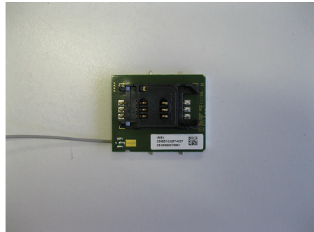
Fig. 11: Telit module - BOTTOM side
