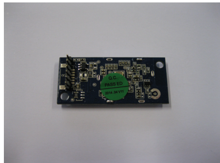
Fig. 13: Sagrad module - BOTTOM side
