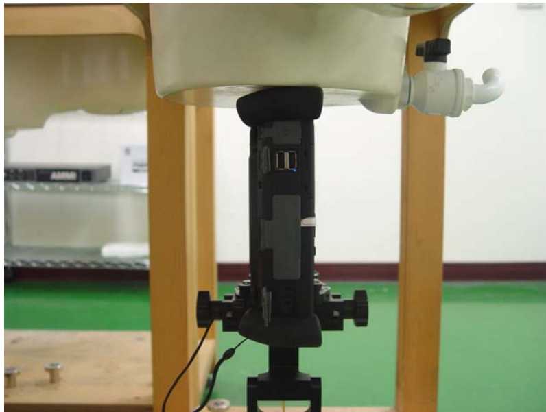
Fig. 9.4 DUT Bottom Side Touch
