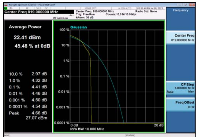
FDD26_Part 90_MidRange_10MHz_819_OneRB_high_Q16
