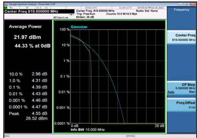
FDD26_Part 90_LowRange_10MHz_819_OneRB_high_Q16
