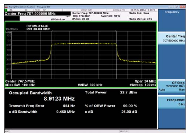
FDD12_MidRange_10_707.5_Q16
