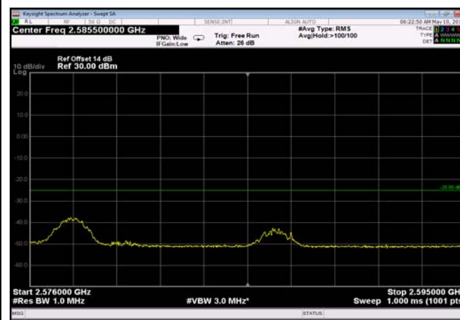
FDD07_20MHz_2560_QPSK_OneRB_low
