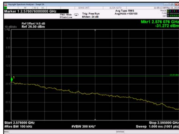
FDD07_20MHz_2560_QPSK_fullIRB_ExtraBan ds_Range_2576~2595 39
