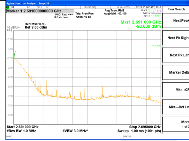
2691-2695MHz
