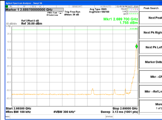
2665-2690MHz
