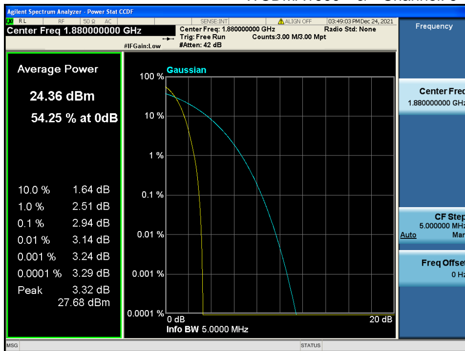
WCDMA1900 & Channel: 9 400
