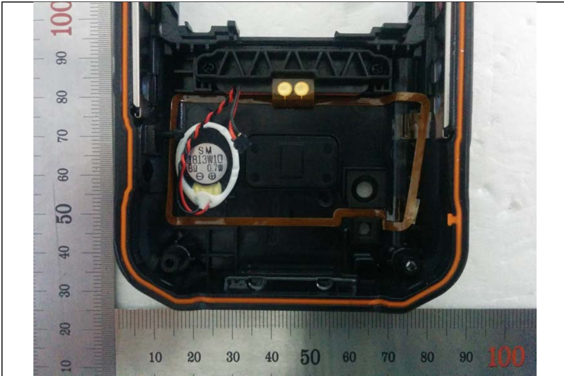
<NFC Antenna>
