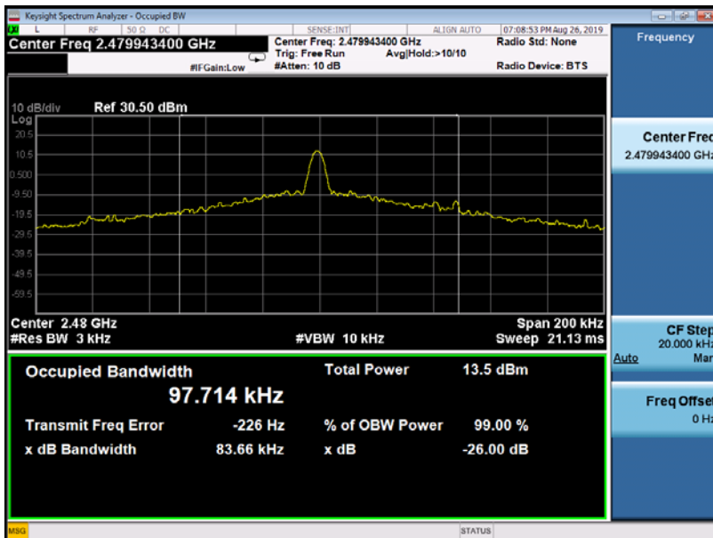
2480MHz
