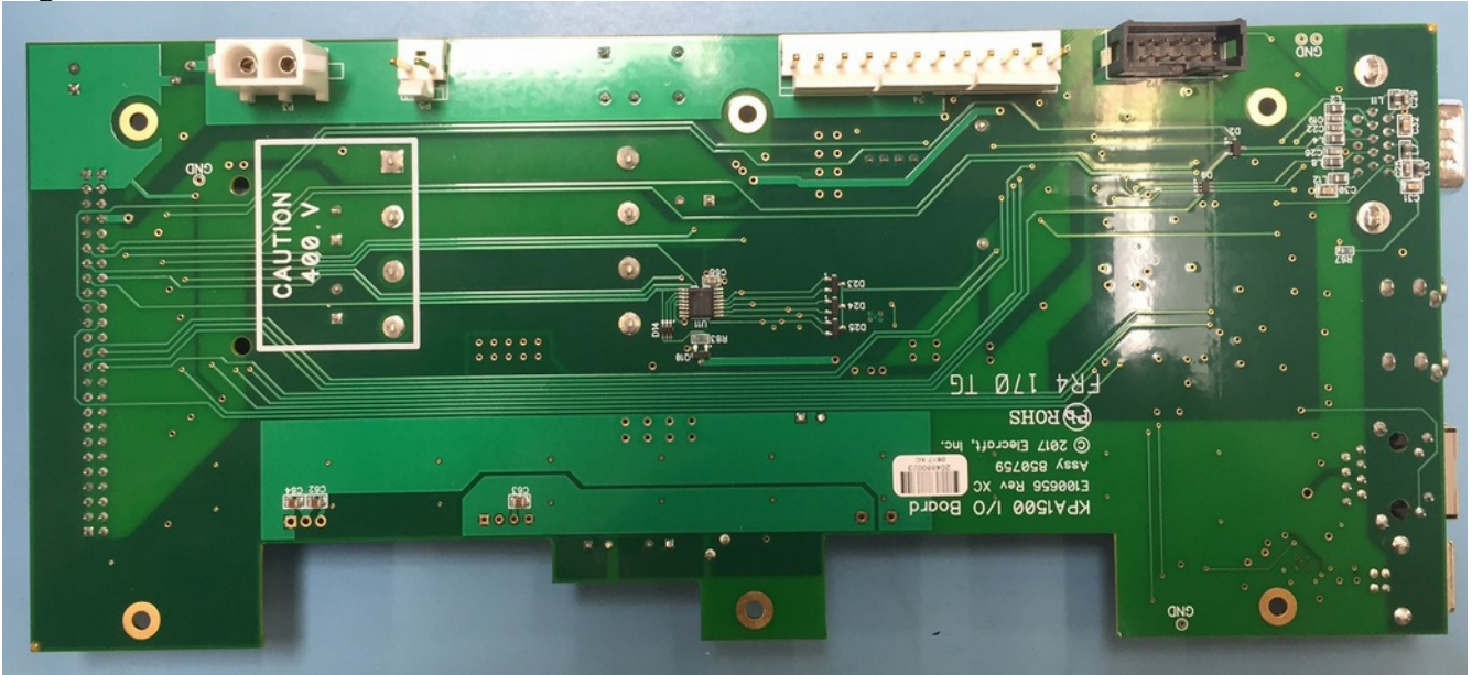
Digital IO Bottom
