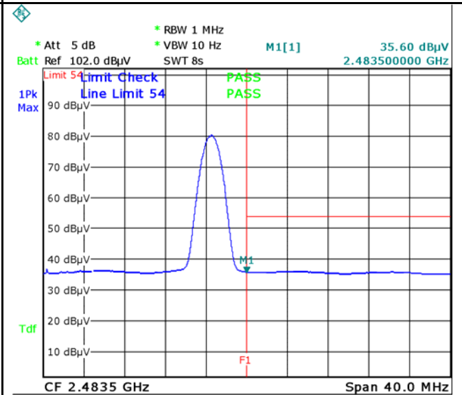
GFSK-Right Side-AV
