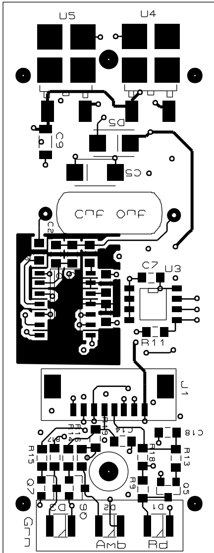
TOP LAYER
