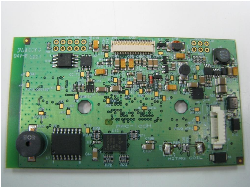
PCB Top
