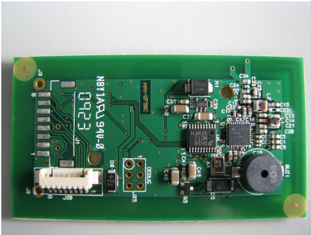
PCB Top
