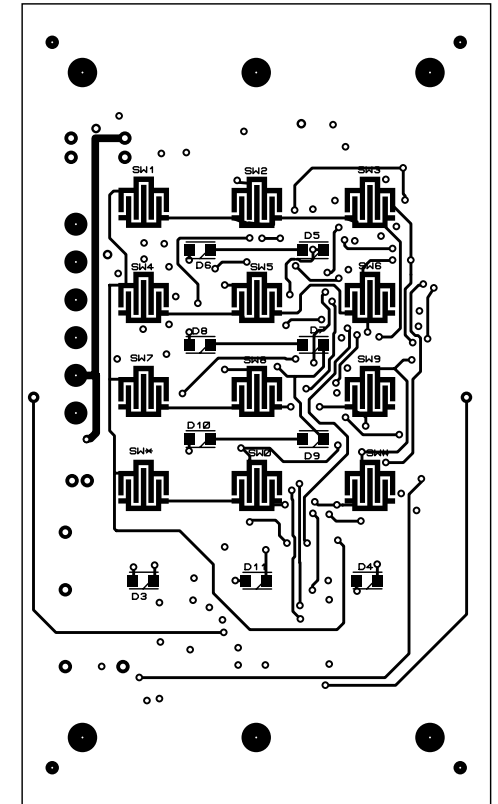
BOTTOM LAYER
