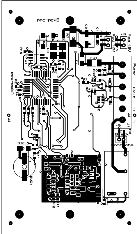
TOP LAYER
