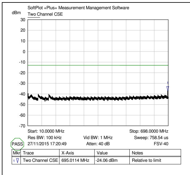
769 - 775 MHz
