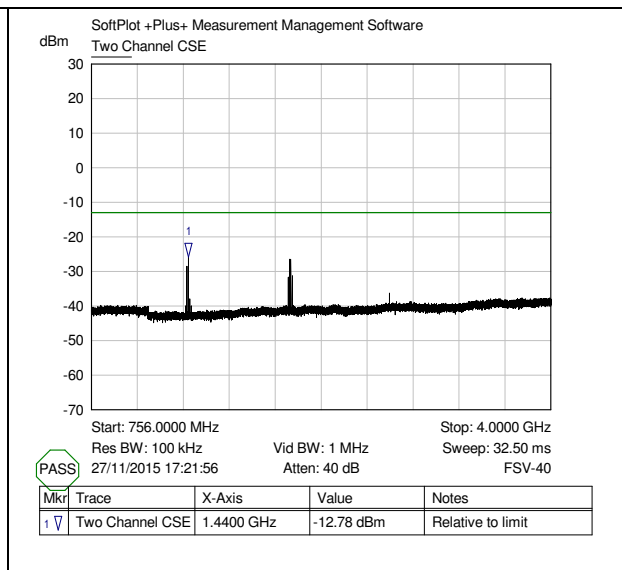
769 - 775 MHz pt 2
