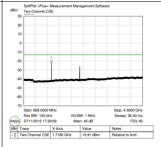
851 - 869 MHz pt 2
