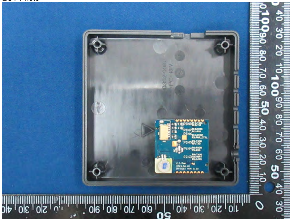
(24) EUT Photo
