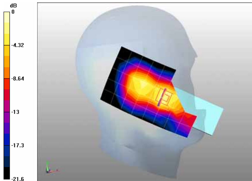
0 dB = 1.46mW/g
