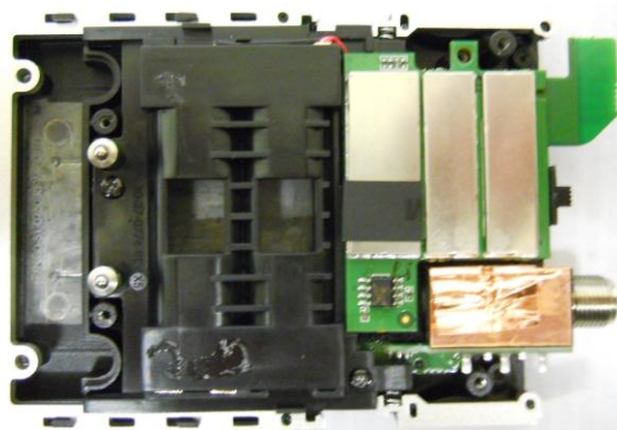
RF PCBA
