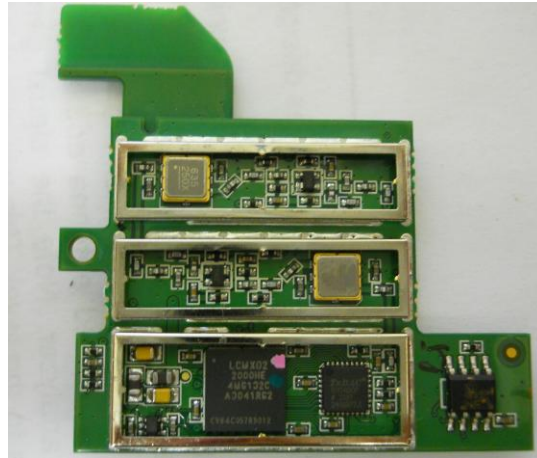
RF PCBA
