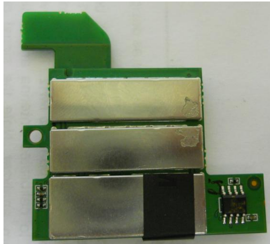
RF PCBA
