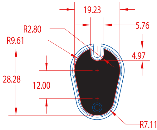
LABEL DIMENSIONS
