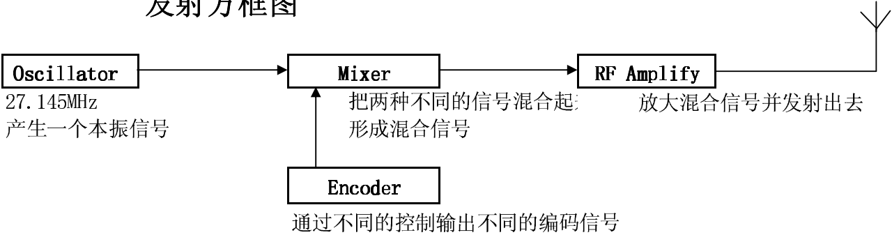
发射方框图
