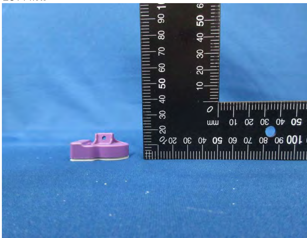
(8) EUT Photo
