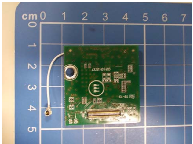
Telit GSM module bottom side
