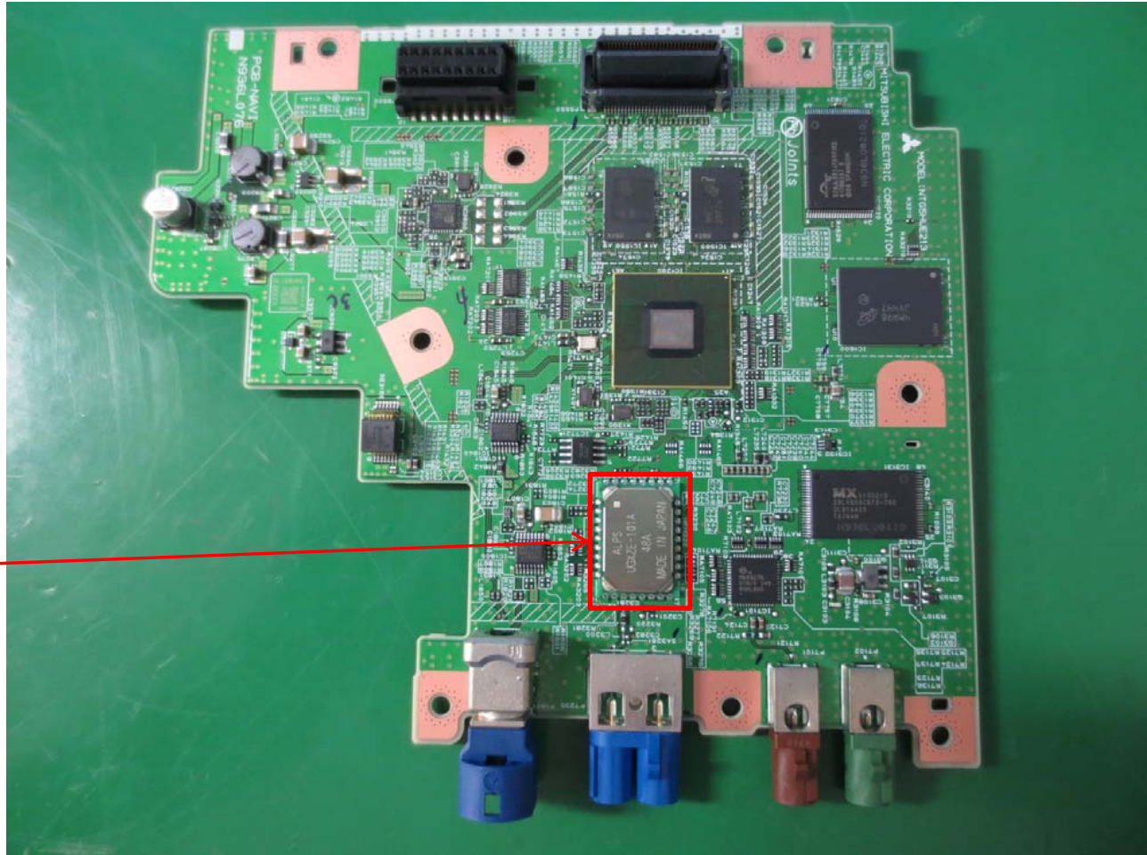
1. PCB-NAVI C-side
