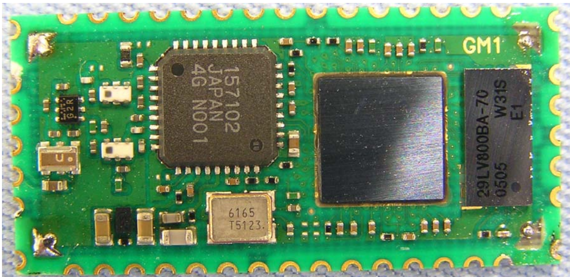
Bluetooth Module Top
