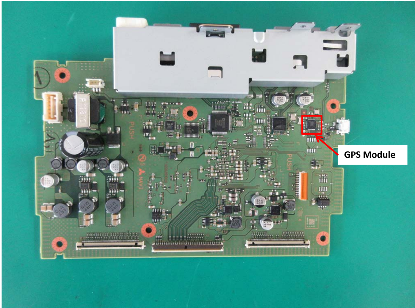
1. PCB-NAVI C-side
