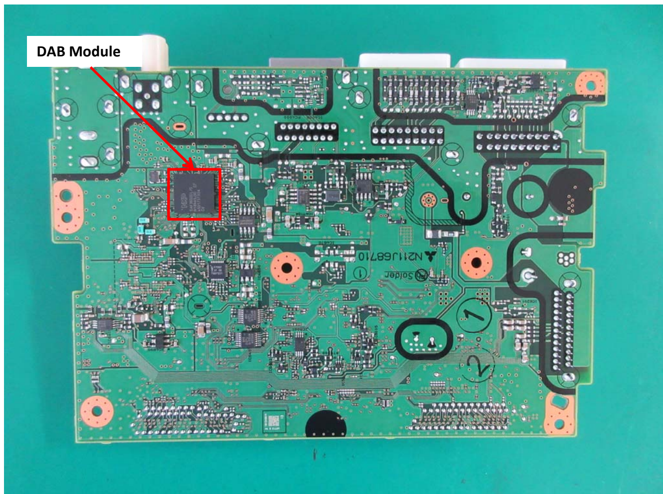
4. PCB-AUDIO S-side
