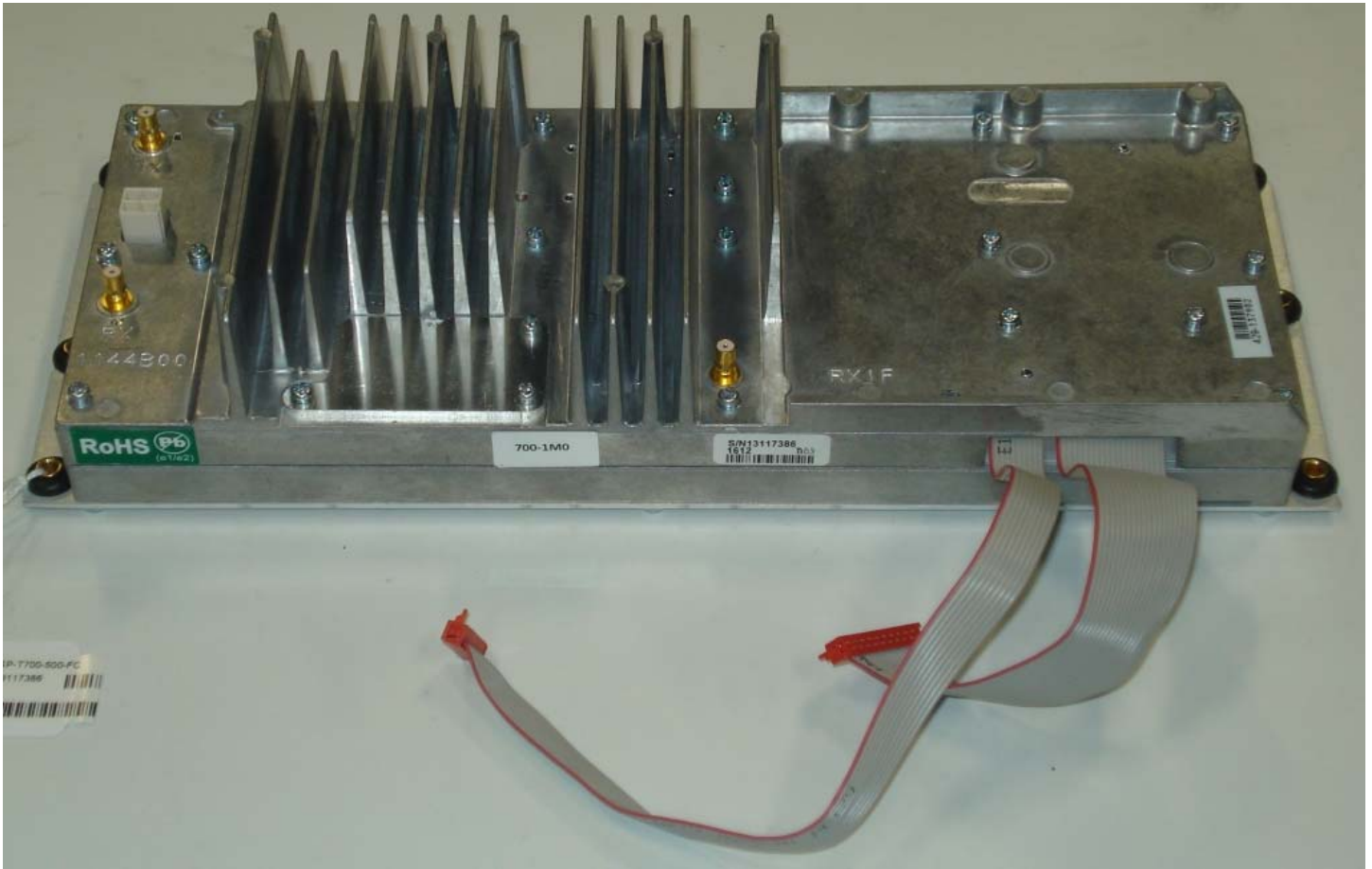
Figure E13.4 – 500kHz RF Module – Front
